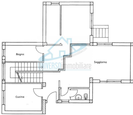
PIANTA PIANO TERRA - Scala 1:50
